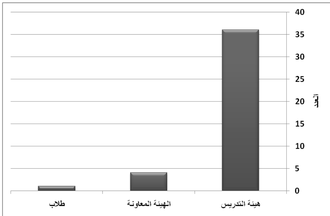
شكل ٣: وظيفة المشاركين في البحث
